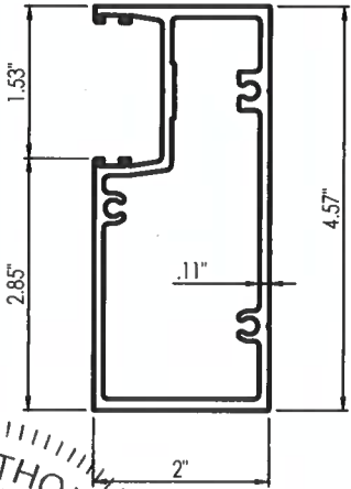
10 FRAME JAMB
